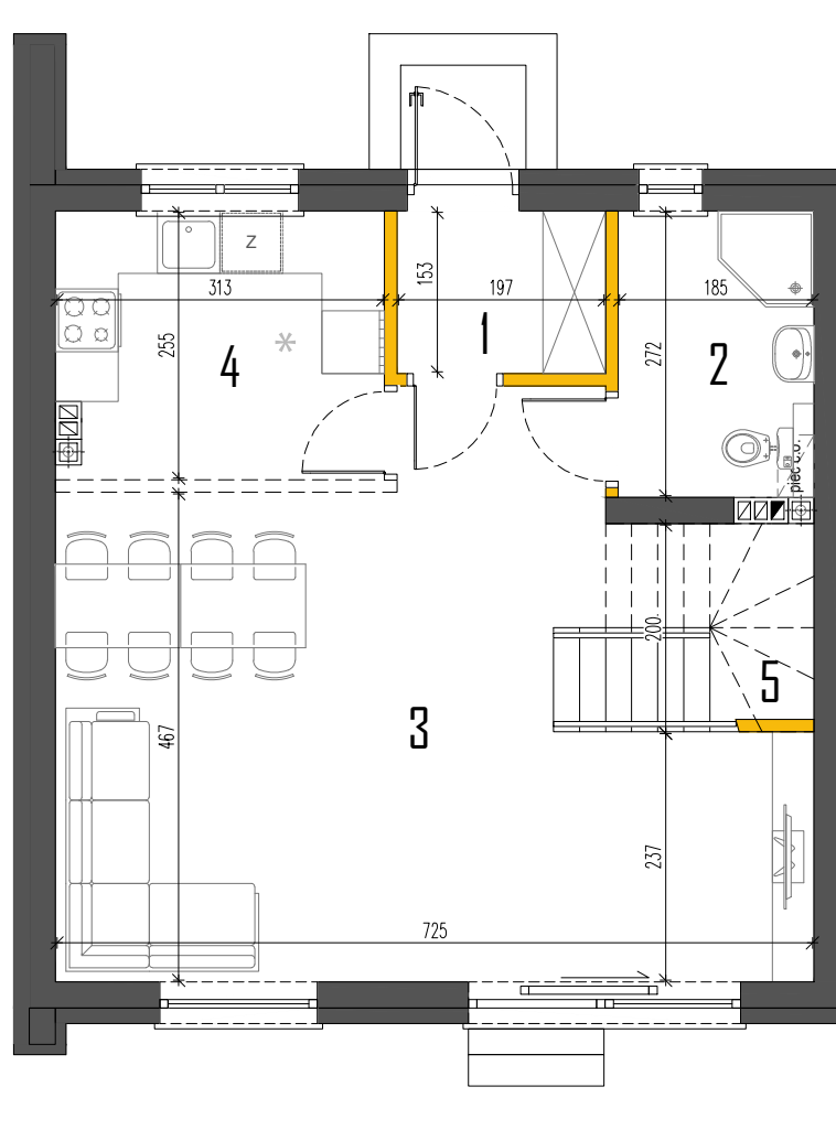
RZUT PARTERU
